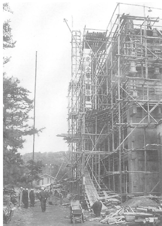
丸太足場の現場をパトロールする京都労研メンバー S. 34. 12
